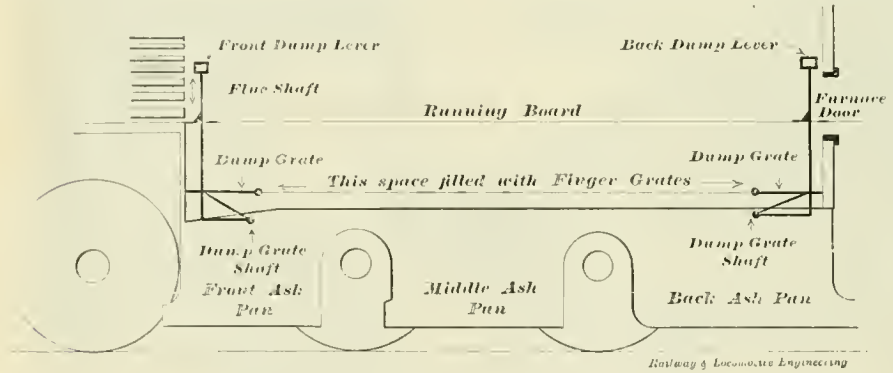
A DUMP GRATE.
